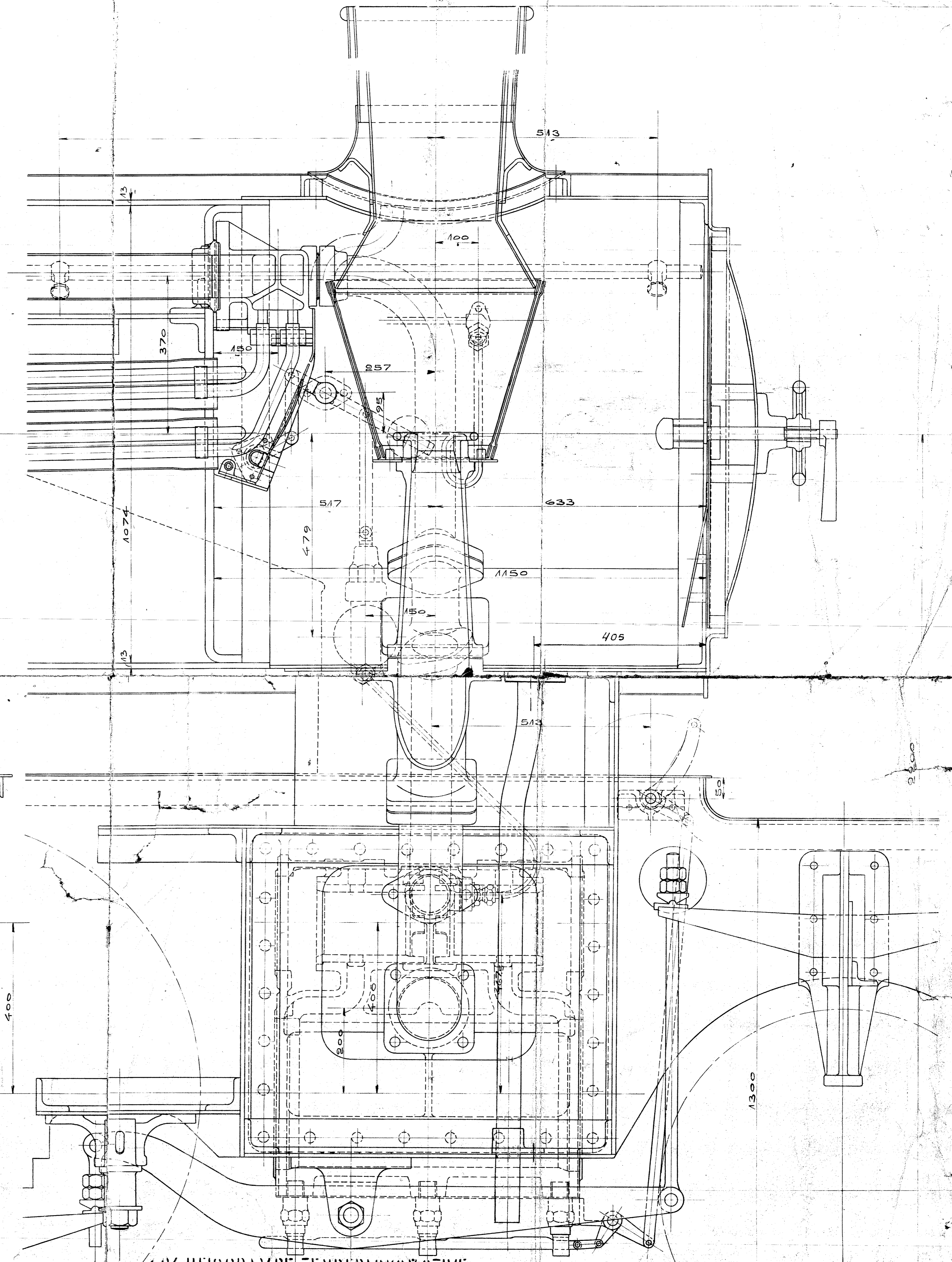
101 HEISSDAMPF-TENDERLOKOMOTIVE FÜR DIE SÜDFRÄNKISCHE EISENBahn. FABRIK № 9983-9986 & 1007-10024. BETRIEBS № 1-7 HENSEL & SOHN. CASSEL 1910
